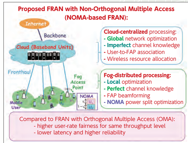
図 クラウド・fog無線アクセスネットワークのための提案 非直交無線資源割り当て法
